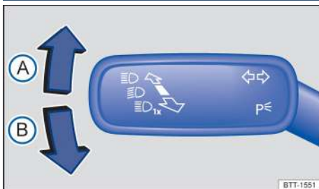
Рисунок 64. Слева от рулевой колонки: Рычаг управления дальним светом и указателя поворота
