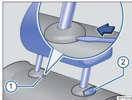
Рисунок 58. Подголовник заднего сиденья: снятие
