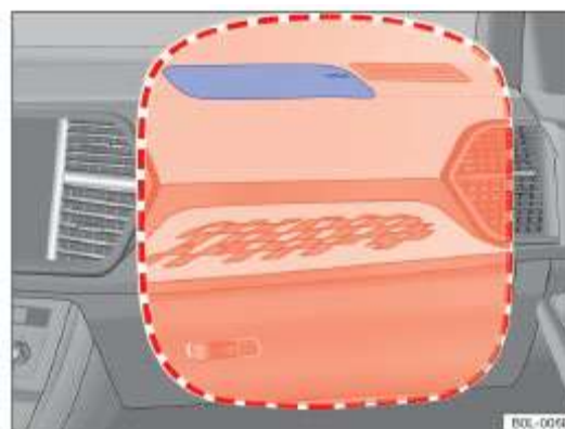
Рисунок 27. Положение установки и диапазон срабатывания фронтальной подушки безопасности переднего пассажира
