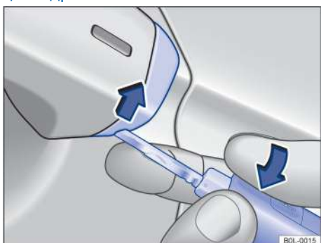
Рисунок 43. Ручка водительской двери: снятие накладки
