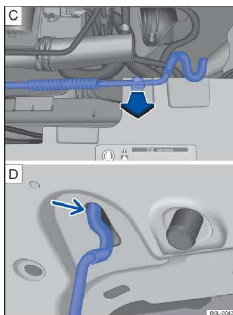
Рисунок 132. С В моторном отсеке: опорный стержень капота моторного отсека в кронштейне; Д На капоте моторного отсека: держатель для опорной штанги капота моторного отсека
