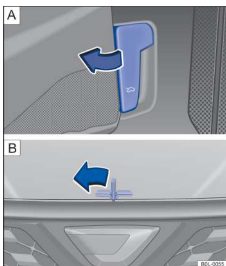
Рисунок 131. А В пространстве для ног со стороны водителя: рычаг отпирания капота моторного отсека; Б рычаг разблокировки в решетке радиатора для открывания капота моторного отсека
