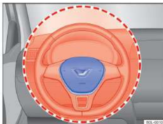
Рисунок 26. Положение установки и диапазон срабатывания фронтальной подушки безопасности водителя
