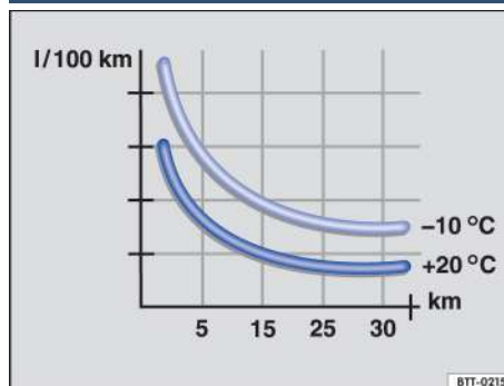
Рисунок 79 Расход топлива на 100 км (л/100 км) при двух разных температурах окружающей среды
