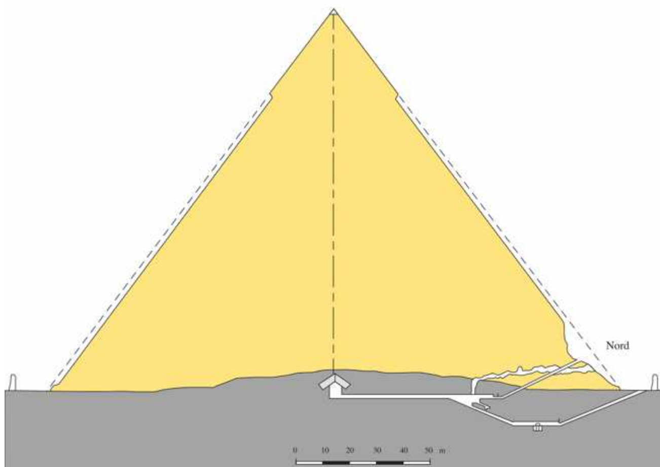
Поперечный разрез пирамиды Хефрена.
