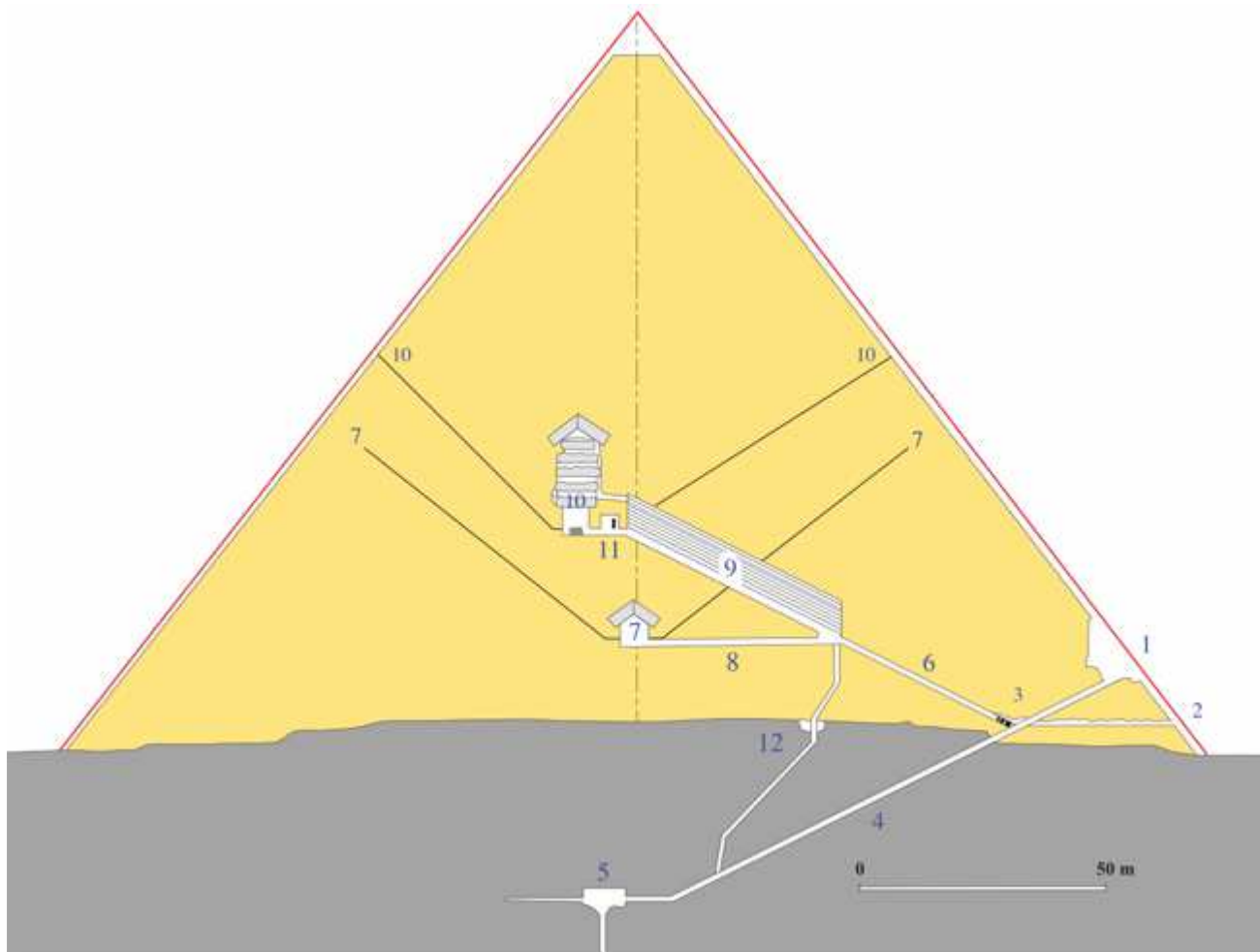
Поперечный разрез пирамиды Хеопса:
