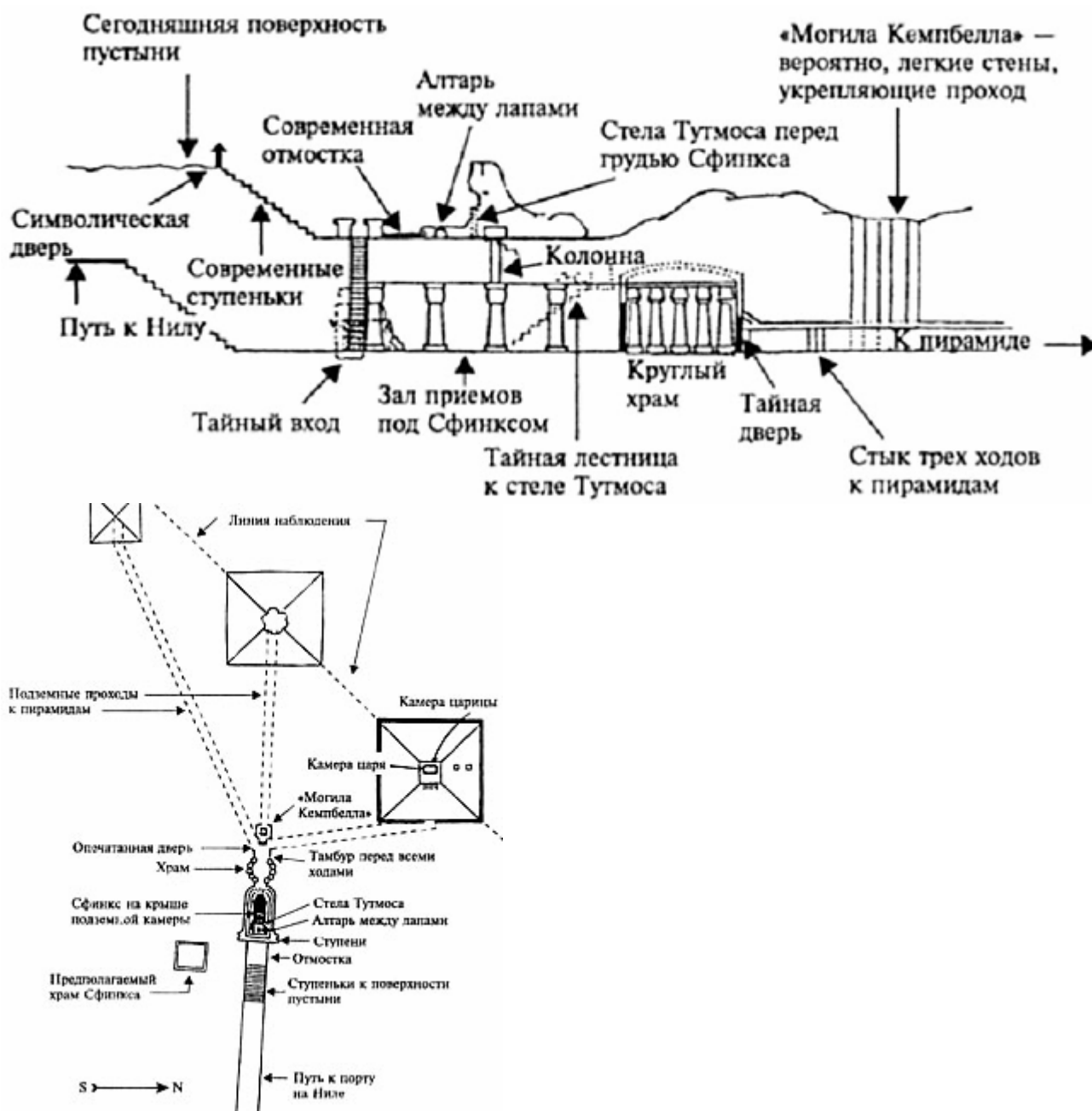
Подземные сооружения в Гизе.
