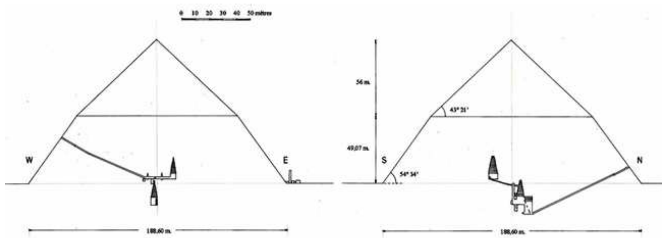
Структура пирамиды.
