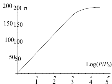
Рис. 3.5. Зависимость степени сжатия \sigma воздуха от давления P .
