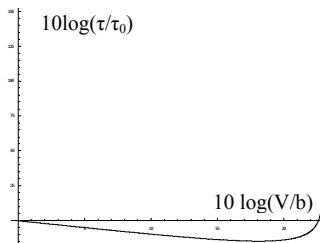
Рис. 3.4. Зависимость времени жизни света в газе от степени его сжатия.
