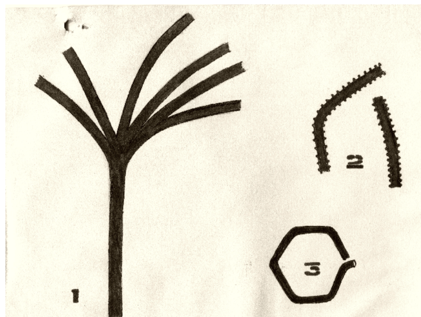
Рис. 13. Зарисовки различных ходов илоедов (1—2) и их слепков (3) в теле и на подошве флишевых ритмов подкотоцкой свиты, палеоцен, Ю. Армения. Натуральная величина.
