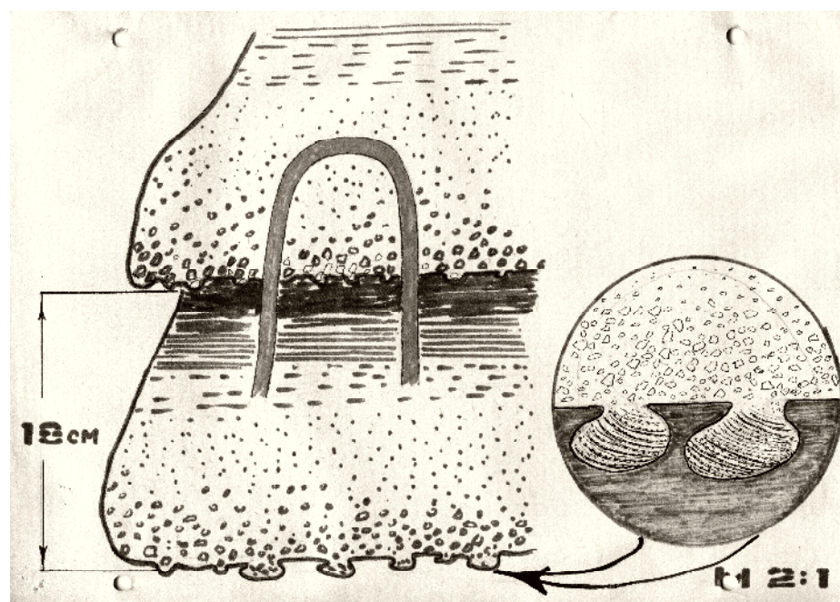
Рис. 14. Ход илоеда — капролит — между двумя флишевыми ритмами в песчаниках подкотоцкой свиты Ю. Армения. На подошве флишевого ритма слепки размыва морского дна, заполненные тонкозернистым пиритом с косо́й слоистостью.
