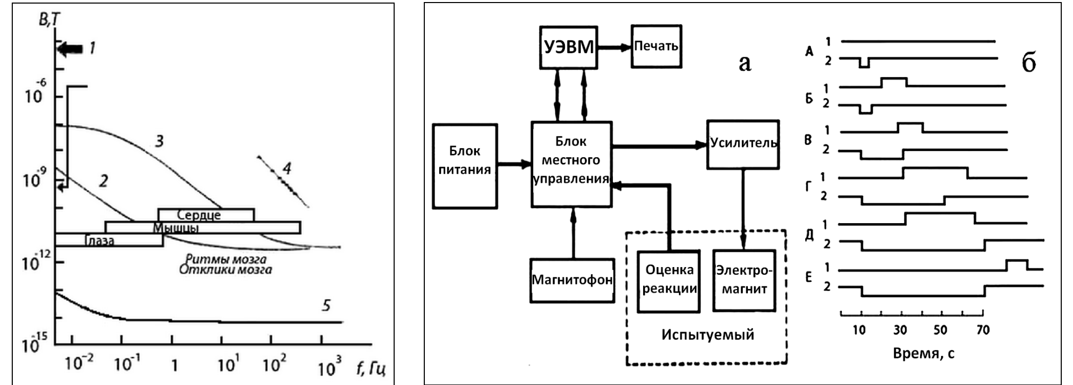
Рис. 15. Спектры биомангнитных сигналов и электромагнитных шумов: 1 — магнитное поле Земли, 2, 3 — геомагнитный и городской шум, 4 — сетевая помеха, 5 — чувствительность сквида [Введенский, Ожогин 1980] Рис. 16. Структурная схема установки эксперимента по магниторецепции ( а ) и реакции испытуемого ( б ) на включение-выключение тока в катушке ( 1 ) ( б ) [Холодов 1982]
