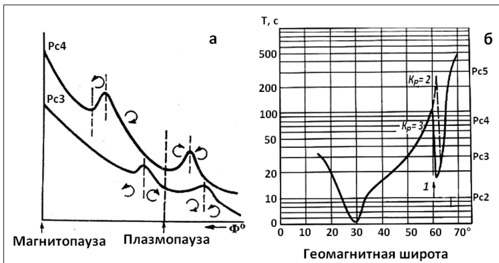
Рис. 12. Геомагнитные пульсации:
