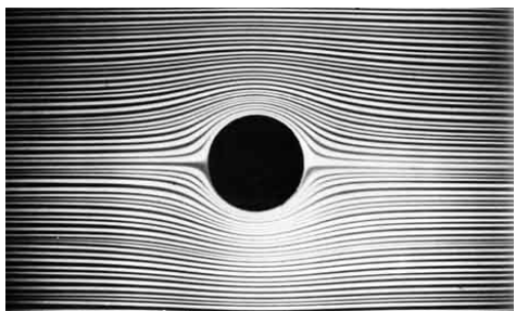
Рис. 43. Ламинарное течение
