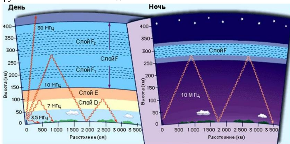
Рис. 2. Схема прохождения электромагнитных волн от коры планеты до ионосферы и сквозь неё.
