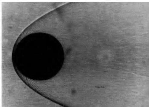
Рис. 5. Шар, движущийся со скоростью M = 7.6 в атмосферном воздухе [71]
