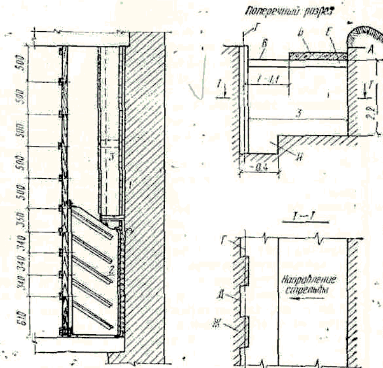
Рис. 4. Пулеулавливатель для стрелкового тира по типовому проекту 294-6-1/74 (вид сбоку):
