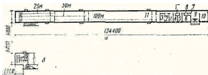
Рис. 11. План закрытого тира по типовому проекту № 294-6-2
